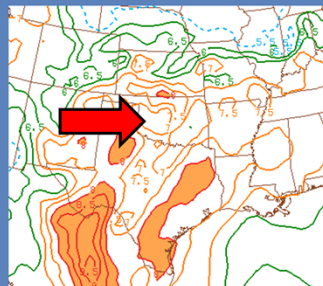
MLLR: 7-7.5°C/km
